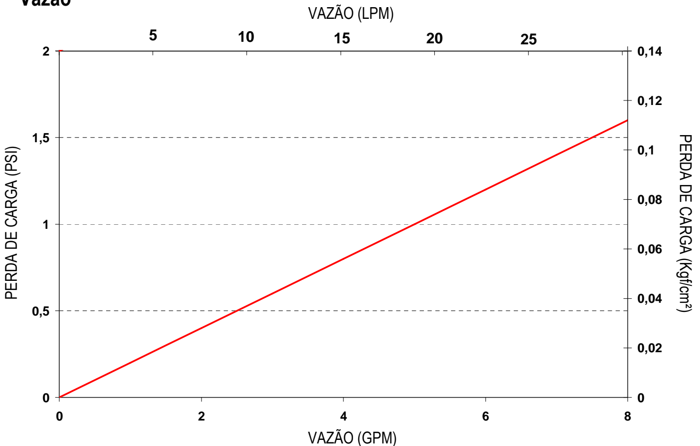
Gráfico: Vazão x perda de carga (água @ 25°C por cartucho de 10").
